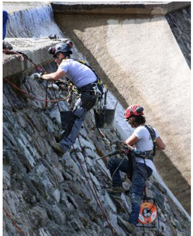
Travaux de rejointoyage du parement aval du grand barrage
